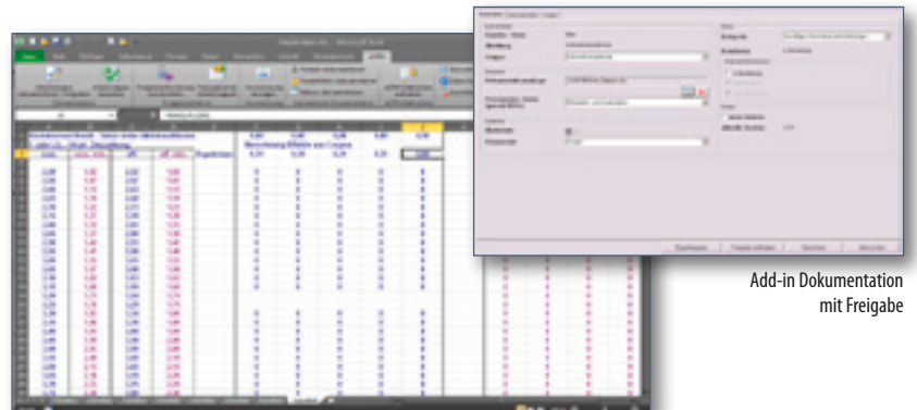
Excel-Ansicht aOPM
